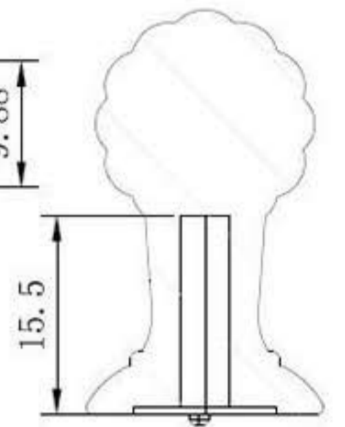
SECTION A-A
