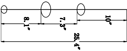
CRS39853PCJ*2PCS L: 25.39"
